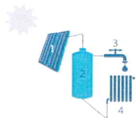
1 Zonnecollector | 2 Opslagvat zonneboiler 3 Sanitair warm water | 4 Afgiftesysteem (radiator, vloerverwarming, etc.)
