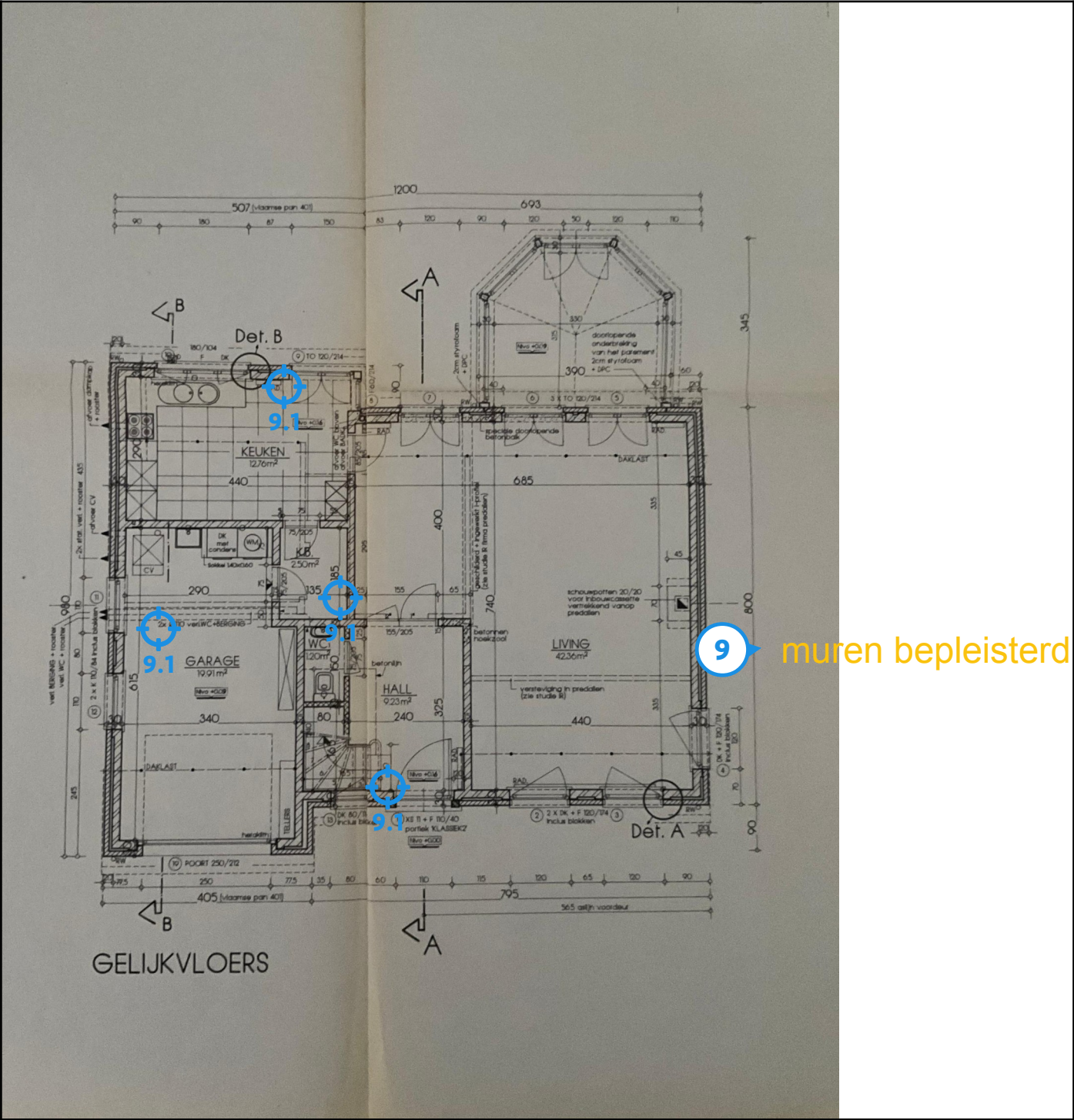
Legende van plan 1.1: Plan Gelijkvloers wanden
