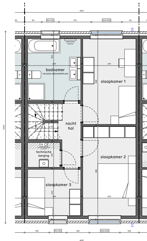
GRONDPLAN verdieping
