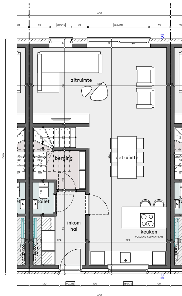
GRONDPLAN gelijkvloers
