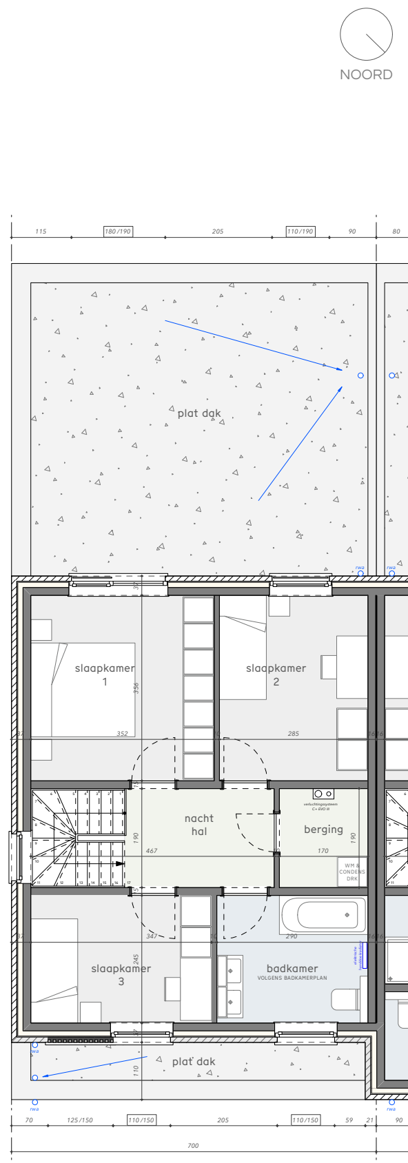
grondplan verdieping
