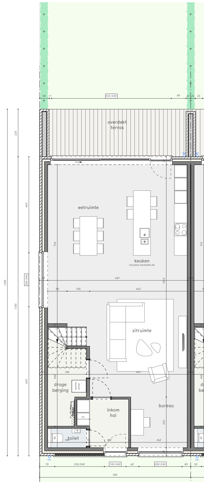
grondplan gelijkvloers
