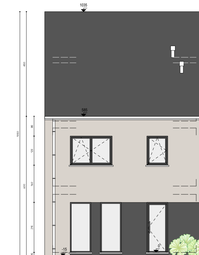
aanzicht voorgevel
