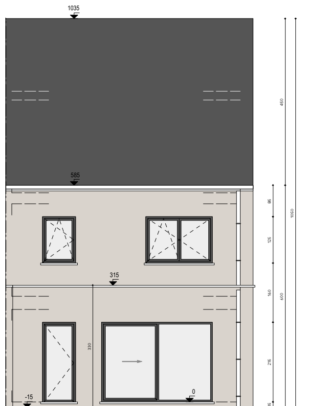
aanzicht achtergevel
