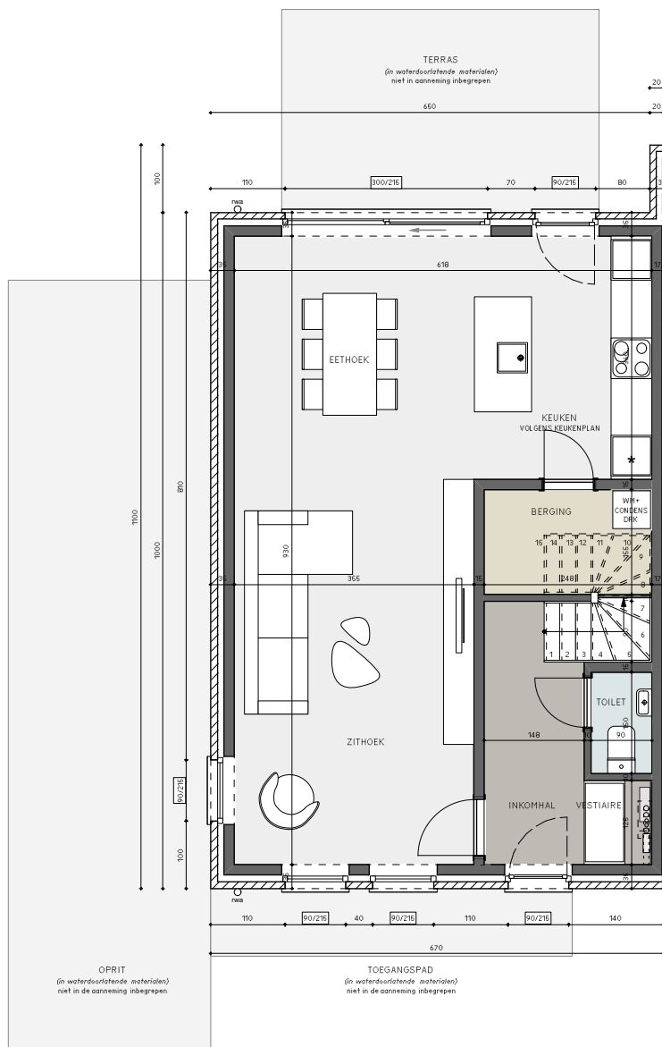
grondplan gelijkvloers
